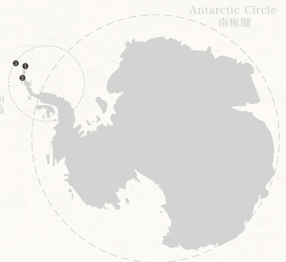
Antarctic Peninsula 南極半島
